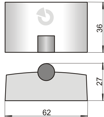
figura: dimensiones del indicador JA-111I.
