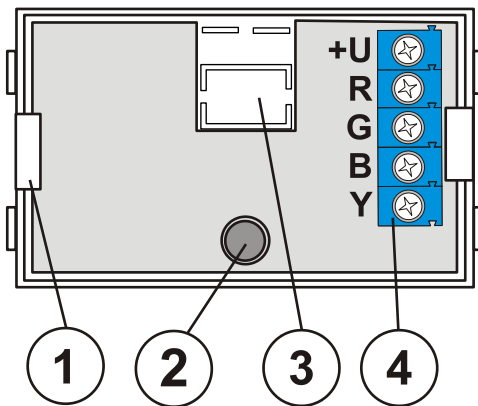
Figura: 1 – fijador de placa; 2 – luz LED; 3 – orificios despegables para pasar el cable; 4 – terminal
