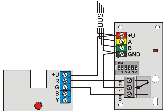
figura: ejemplo de conexión para indicación bicolor del estado de salida PG
