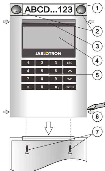
Figura: 1 - segmento de mando; 2 - botones retroiluminados; 3 - botón de activación retroiluminado; 4 - pantalla LCD de información; 5 - módulo de acceso con RFID lector; 6 - cerrojos de apertura del módulo; 7 - tornillos de la tapa del teclado
