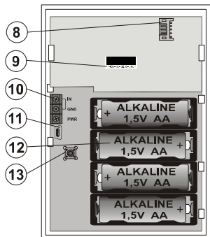
Figura: 8 - conector para la conexión del primer segmento de mando; 9 - número de serie; 10 - caja de bornes; 11 - conector mini USB; 12 - pilas; 13 - conmutador de sabotaje
