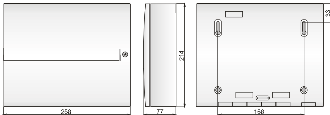
Dimensiones de la caja
