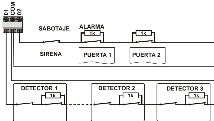
Máximo 5 detectores en un lazo
